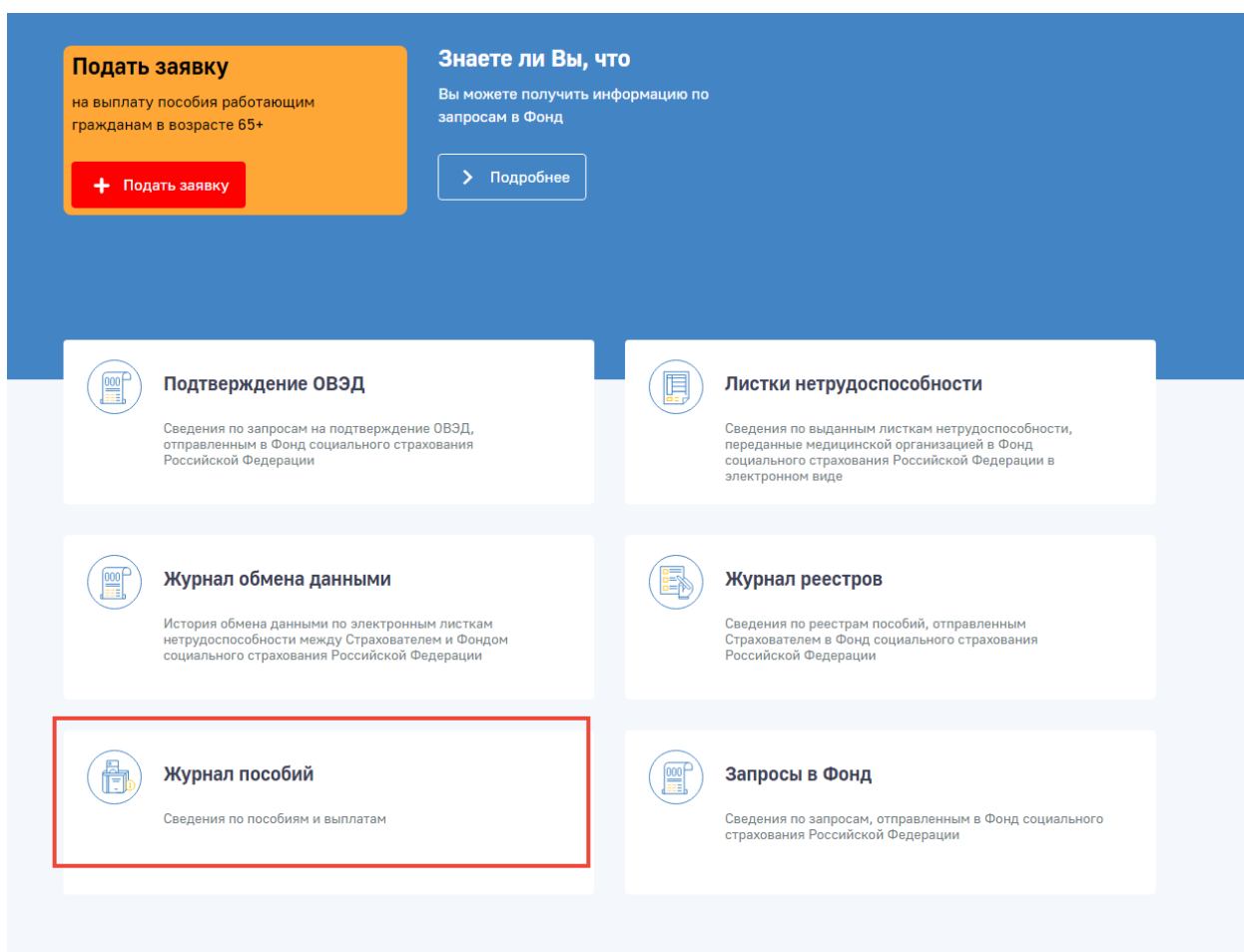
Рисунок 3 – Журнал пособий
